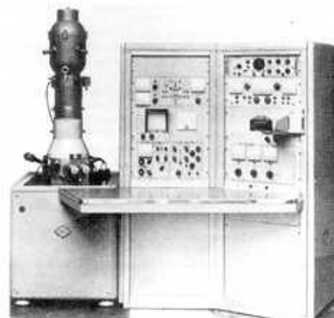
PRVNÍ SÉRIOVĚ VYRÁBĚNÝ RASTROVACÍ MIKROSKOP 1965
