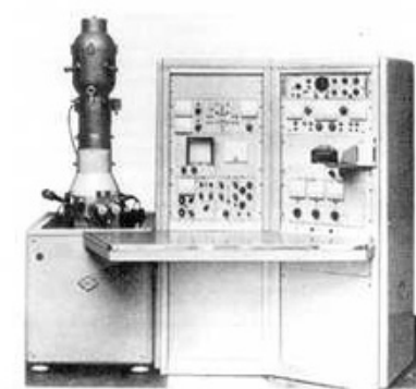
PRVNÍ SÉRIOVĚ VYRÁBĚNÝ RASTROVACÍ MIKROSKOP 1965
